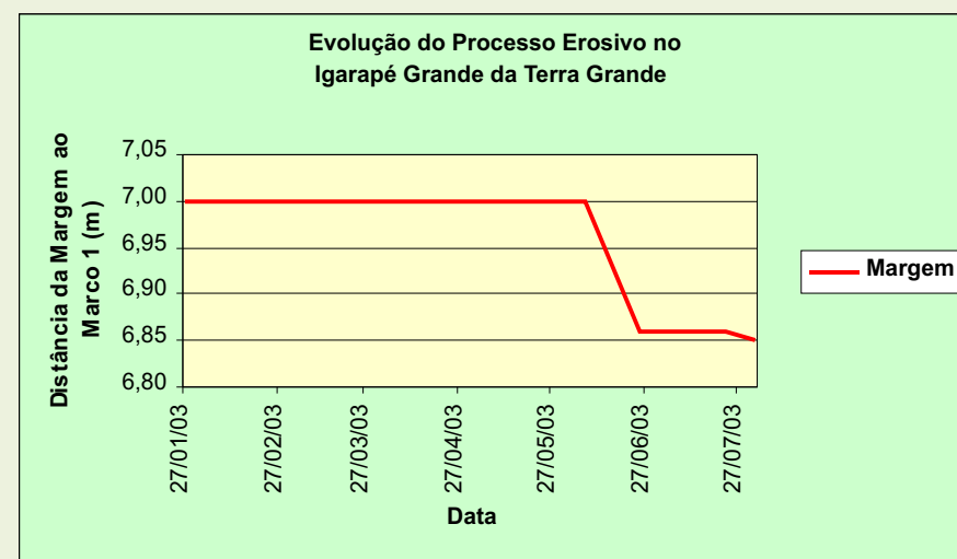
MEDIÇÕES REALIZADAS NO MARCO 1
