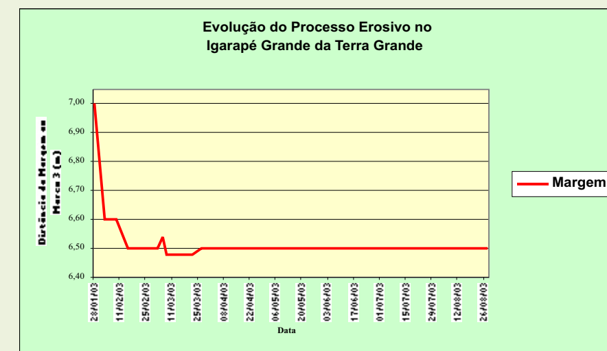
MEDIÇÕES REALIZADAS NO MARCO 3
