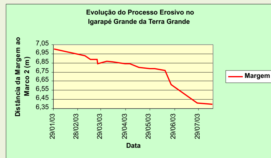
MEDIÇÕES REALIZADAS NO MARCO 2
